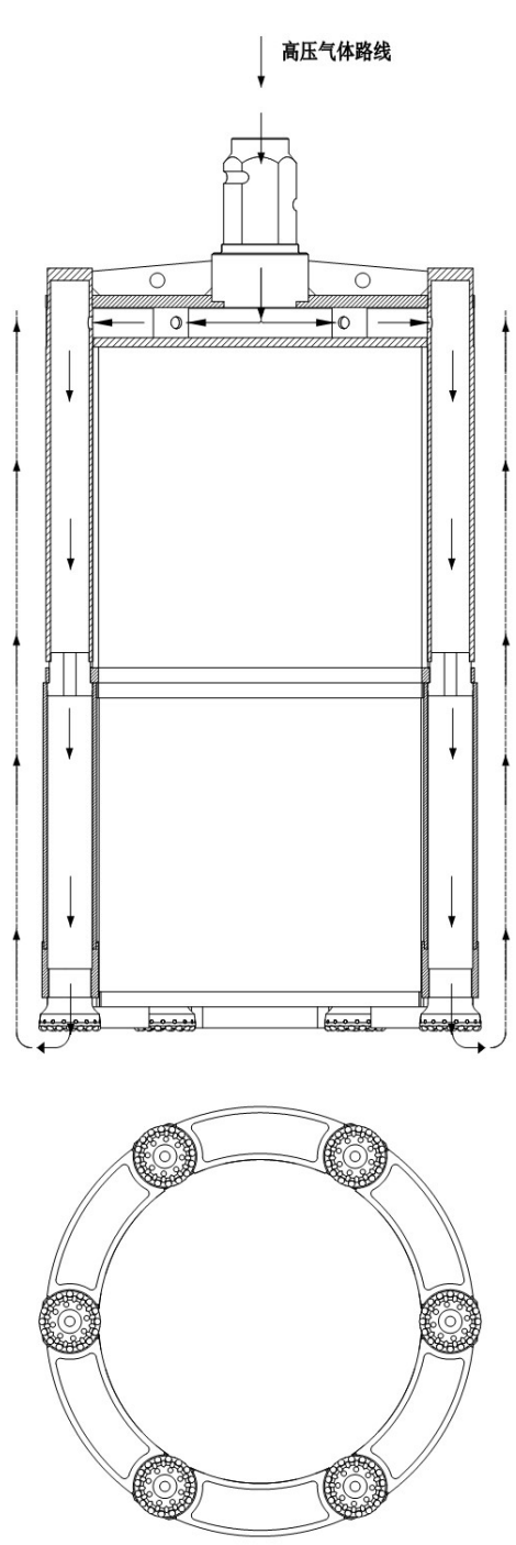
图 3 环切型集束式潜孔锤
