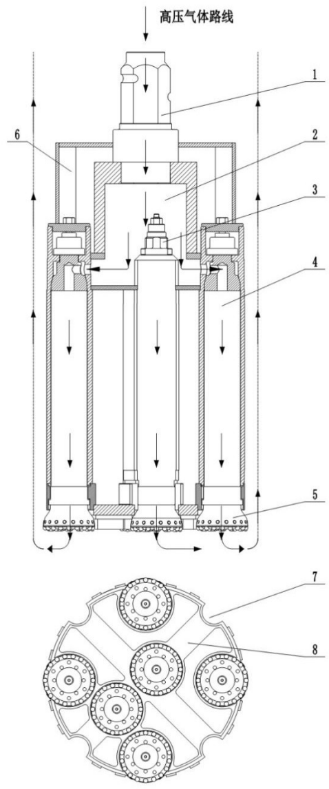
1. 接头 2. 气体分配腔 3. 紧固装置 4. 潜孔冲击器 5. 潜孔钻头 6. 锤体上盖 7. 锤体排渣通道 8. 锤体
