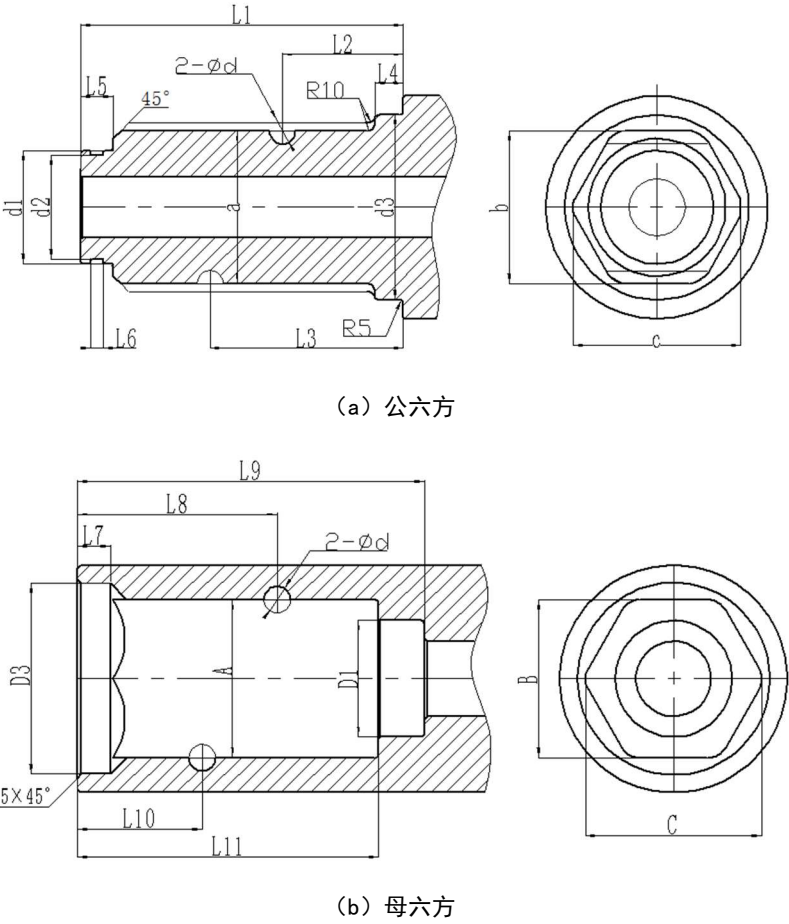
图 6 六方接头
