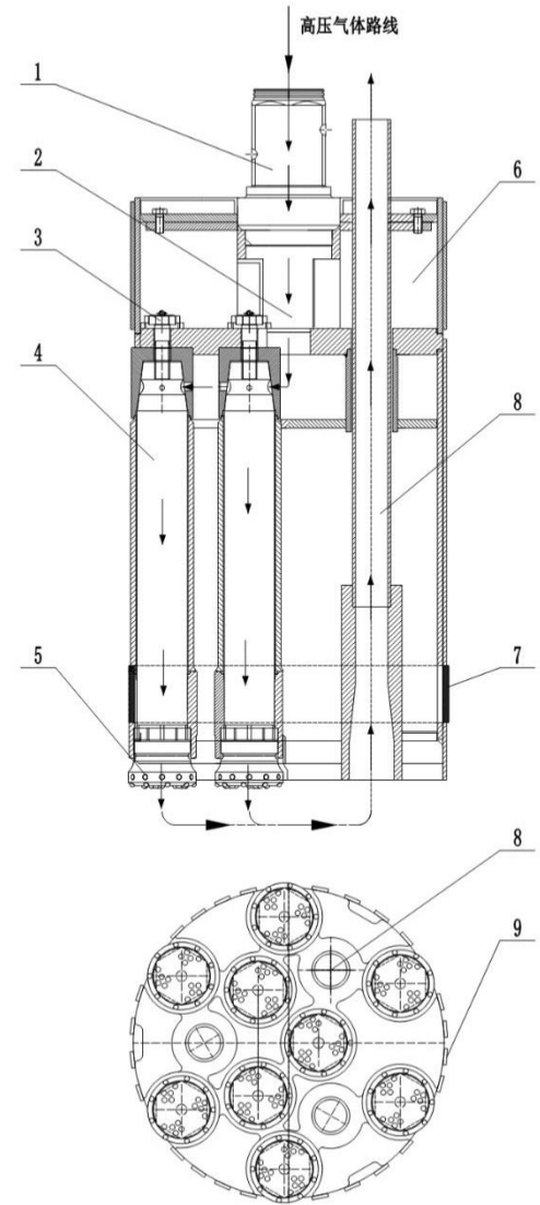
1. 接头 2. 气体分配腔 3. 紧固装置 4. 潜孔冲击器 5. 潜孔钻头 6. 锤体上盖 7. 止风环带 8. 排渣管 9. 耐磨条带
